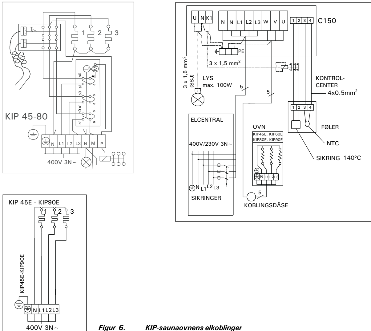
Figur 6. KIP-saunaovnens elkoblinger
