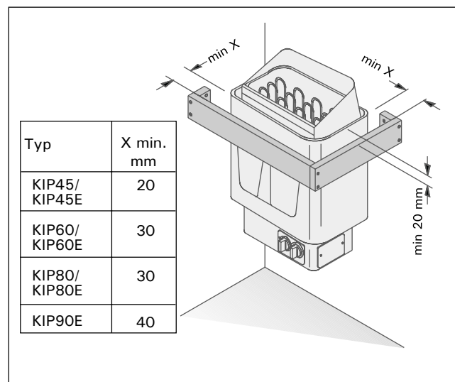
Figur 3. Sikkerhedsgelænder
