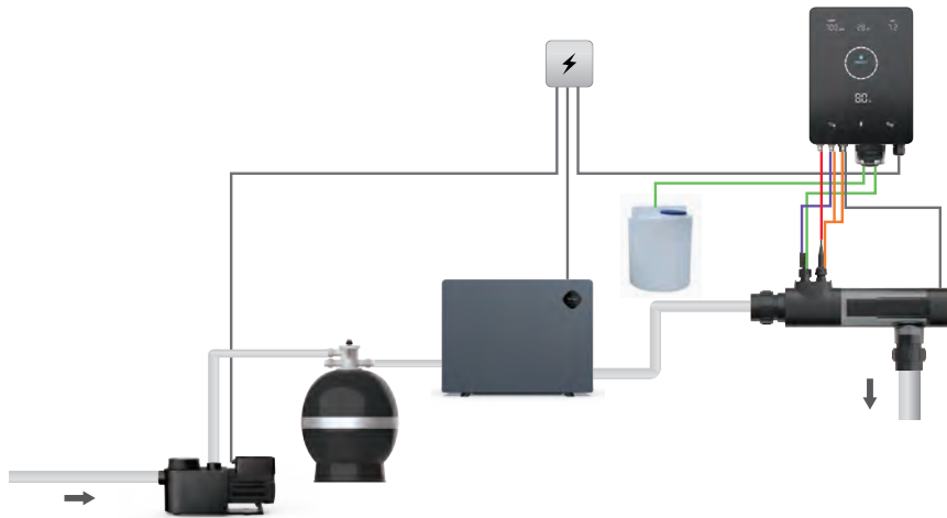
① Installationsschema
