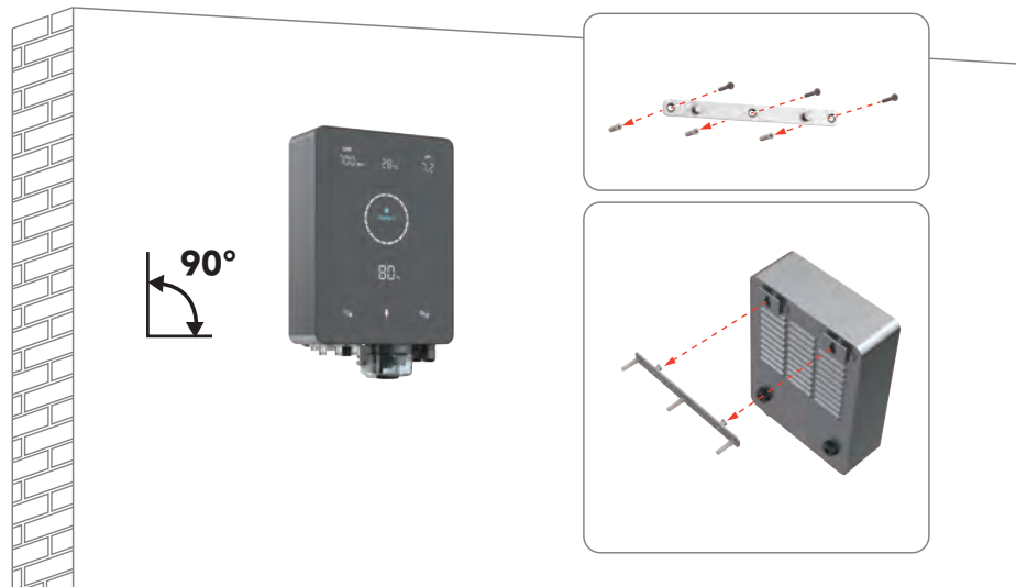
③ Installation av styrenhet
